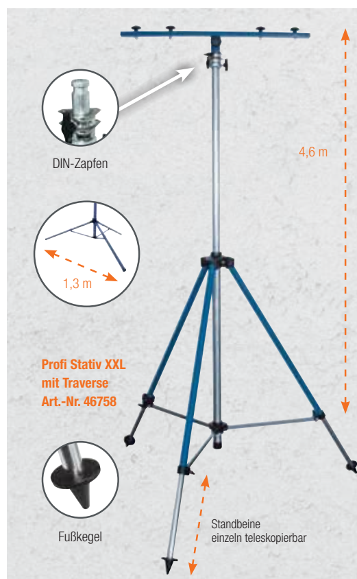
Maße Traverse
